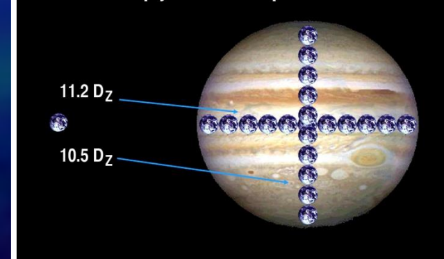
Spljoštenost Jupitera
