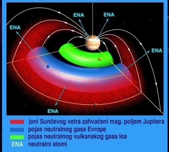
Gradnja Jupiterove magnetosfere
